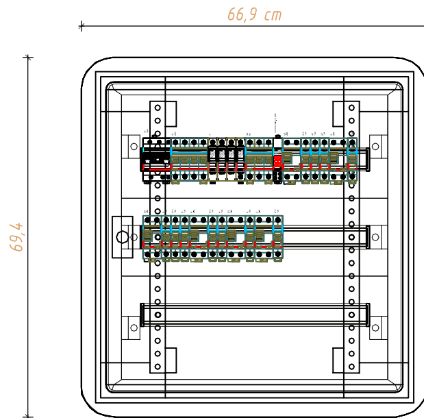
Rozdzielnica wtykowa, izolacyjna, wyposażona, np. XL 3 160, 3x24 mod., drzwiczki płaskie, metalowe, montaż na wysokości ok. 120 cm od posadzki.
